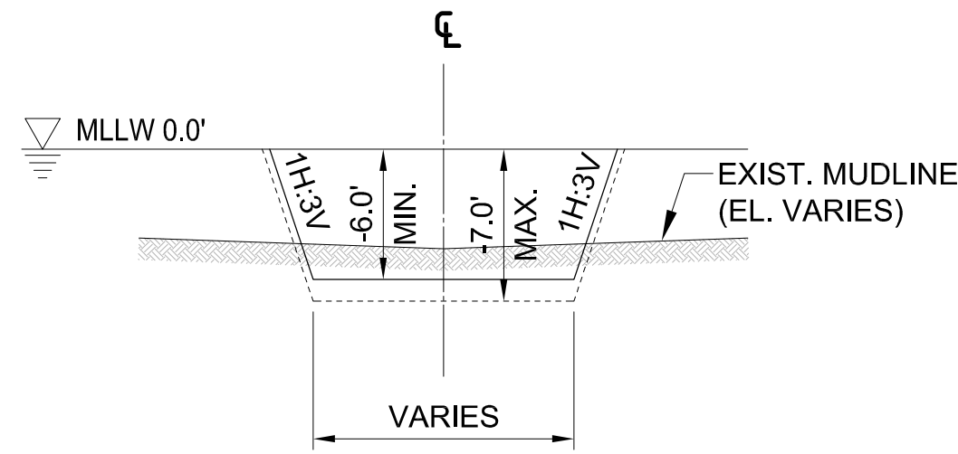
TYPICAL SECTION N.T.S.
